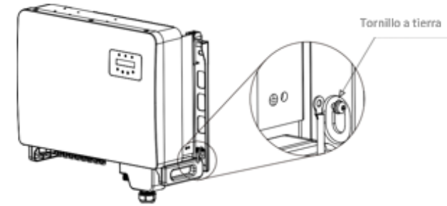
Figura 5.14 Cable fijo
